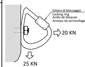
Art. 700 - Mini Top Ø 8 mm + Art. 122 - Hang Fix inox M8L Peso Weight Peso Poids 133 g Hang Fix M 8 x 78 mm
