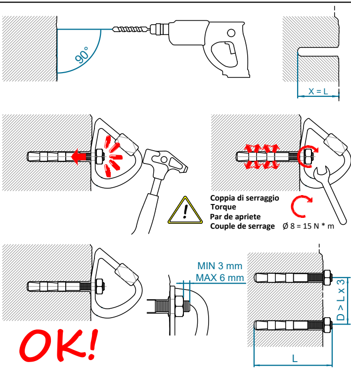
Art. 700 - Mini Top Ø 8 mm Peso Weight Peso Poids 100 g
