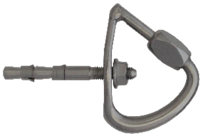
Art. 700 - Mini Top Ø 8 mm + Art. 122 - Hang Fix inox M8L Peso Weight Peso Poids 133 g Hang Fix M 8 x 78 mm
